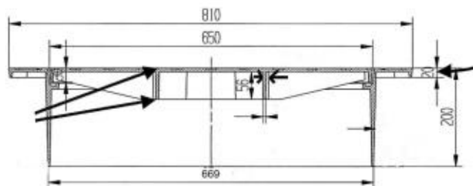
Дождеприемник круглый ДК (D400) плавающий с шарниром с 2-ми замками, с резиновой прокладкой
